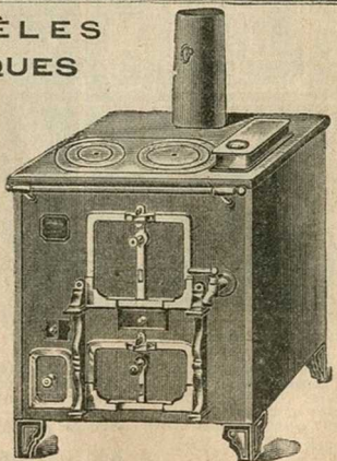
Fourneau "Au Châtelet" en tôle et fonte, à retour de flamme. Long. 0=70, prof 0=45, haut. 0=80
