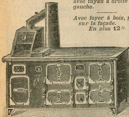
Fourneau 2 fours, 2 étuves, grillade ordinaire et chauffe-assiettes.
