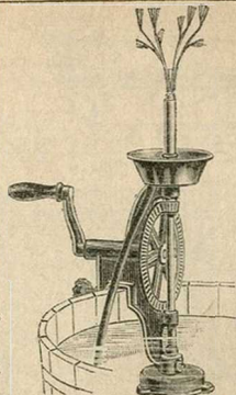
Machine à rincer les bouteilles, modèle léger pour ménage. . 11.90 Modèle soigné renforcé. 22.25
